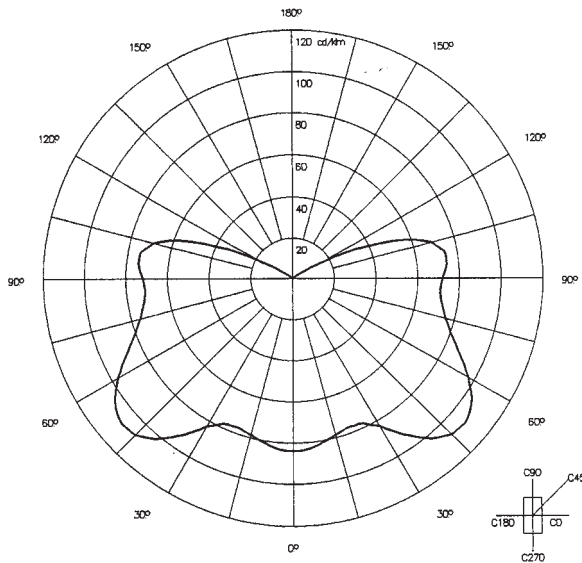
HPS-E 70W
